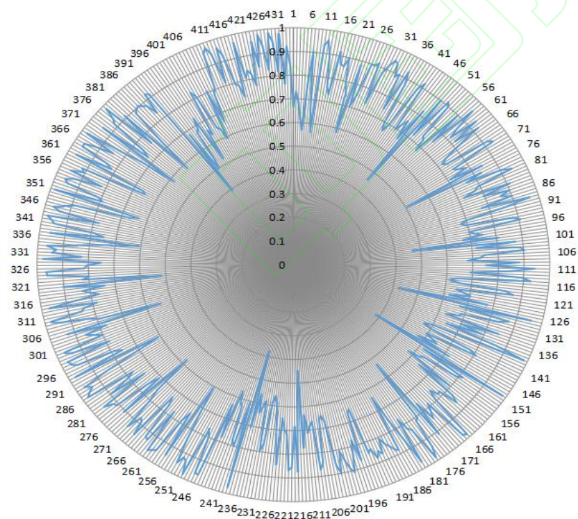
图 3 玄参农残图谱相似度的雷达分布
