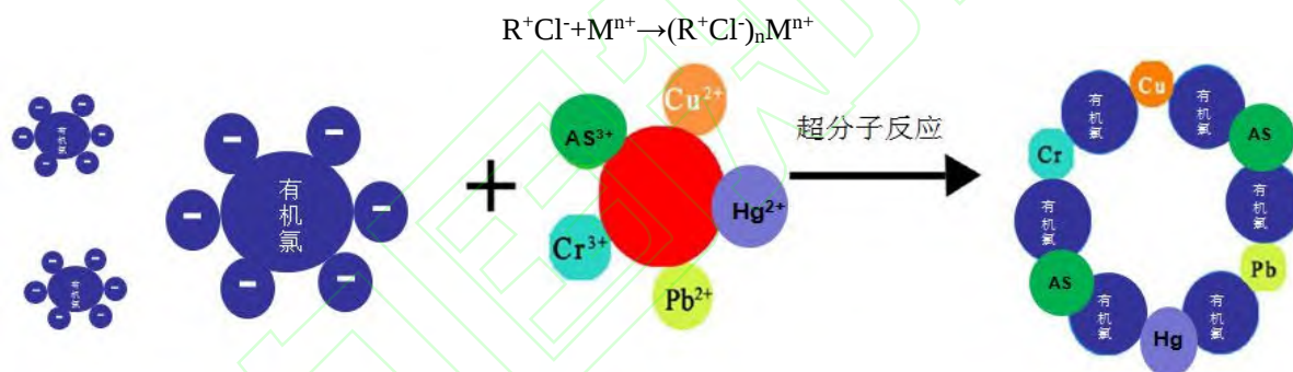
图 1 重金属与农药的超分子结构
